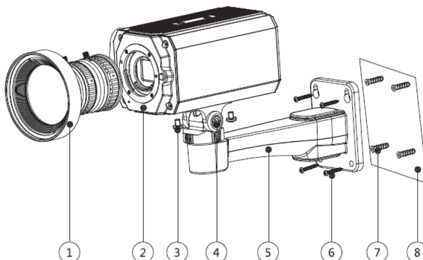
Figure 8-6 Componentes del dispositivo
