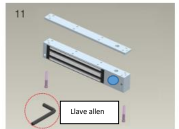
Ajuste los opresores con la llave.
